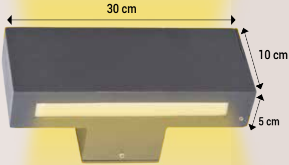
ŞA 3180 Duvar Apliği 10 W SMD LED IP 67 Elektronik Sürücü
